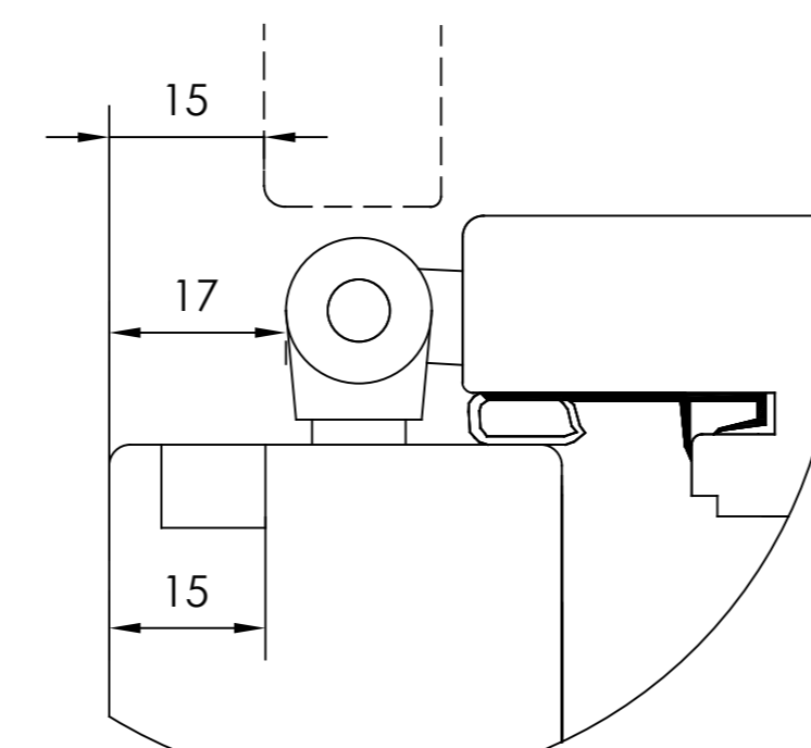
- Utanpåliggande gångjärn
