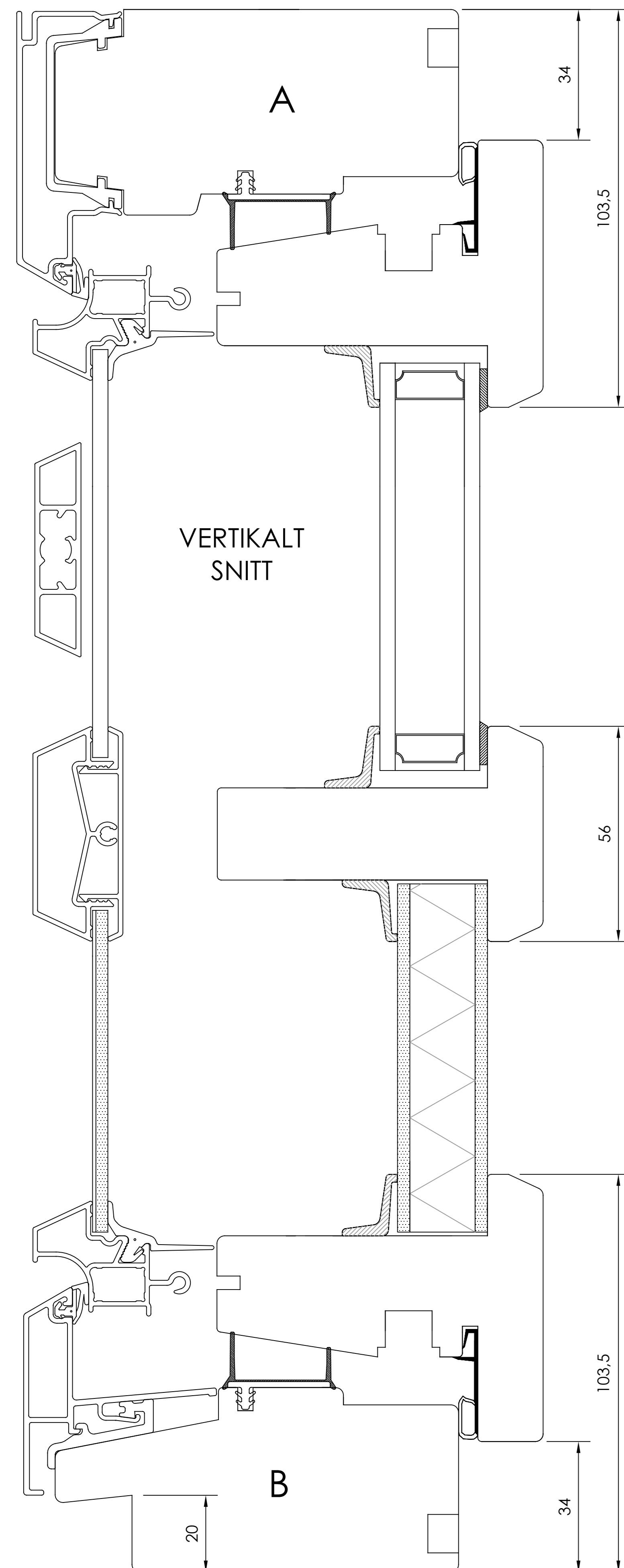
Standard tröskel
