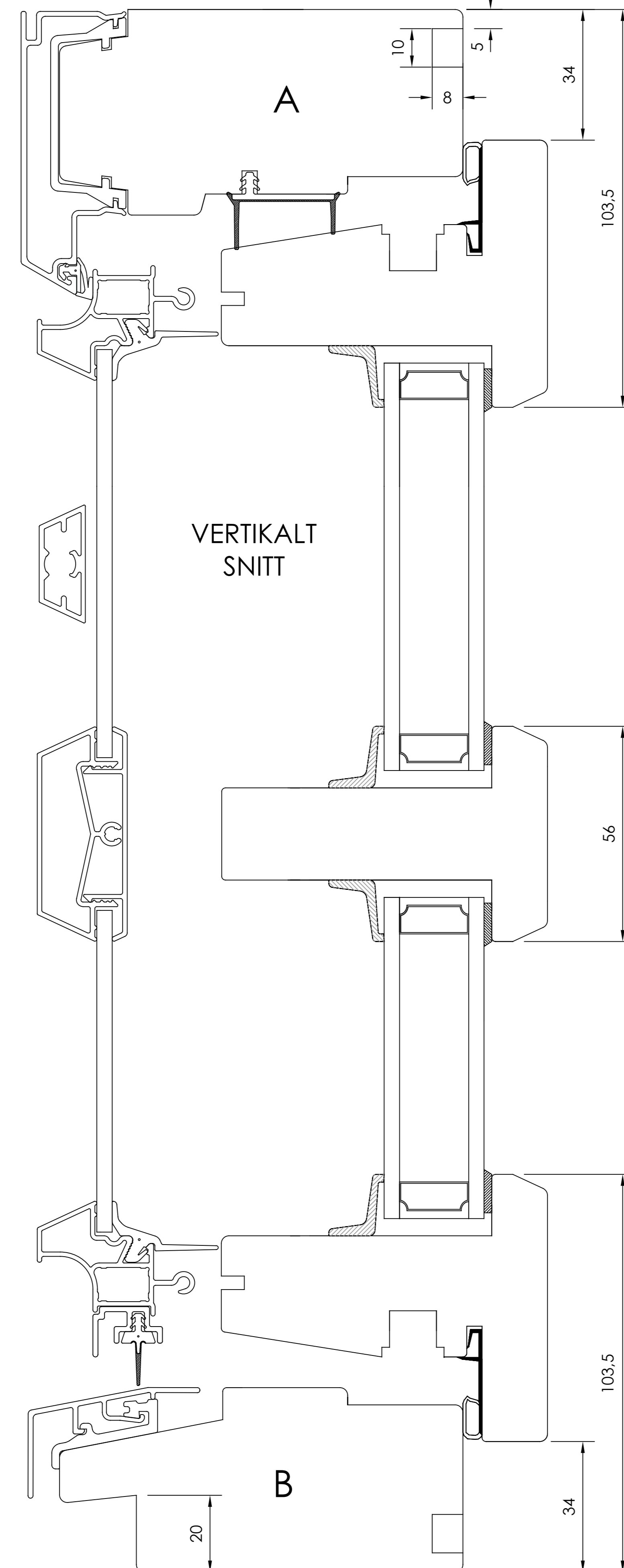
Låg tröskel
